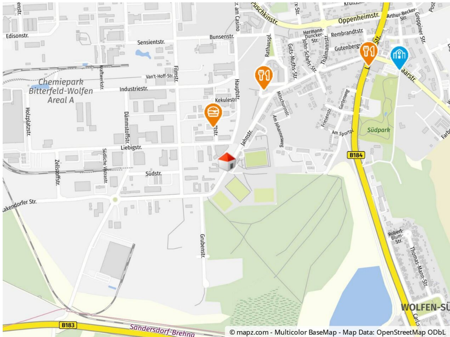
Geolyzer Kartenausschnitt
